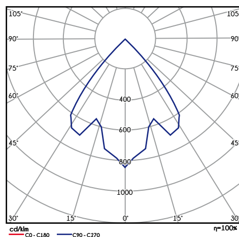
Courbe photométrique d'un luminaire à LED à rendement 100 %
