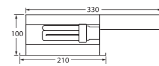
lampe TC-TEL 26 ou 32W
